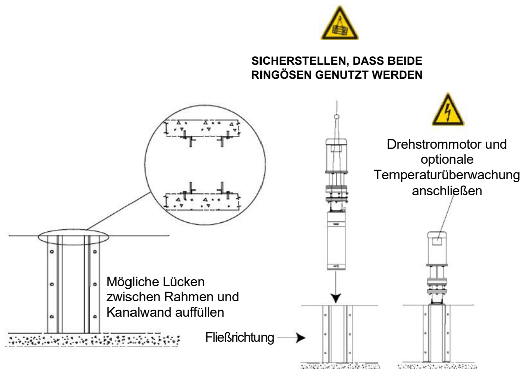
Installation des Zerkleinerers
