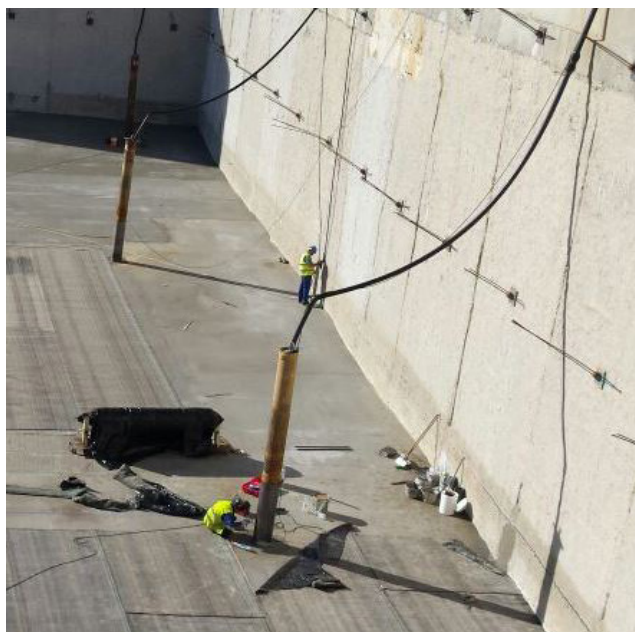
Instalación de los pozos de drenaje y las bombas de achique
