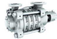
MBN 节段式多级泵
