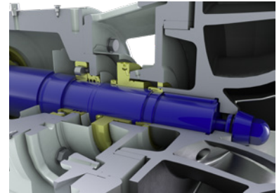
Garniture mécanique à cartouche
