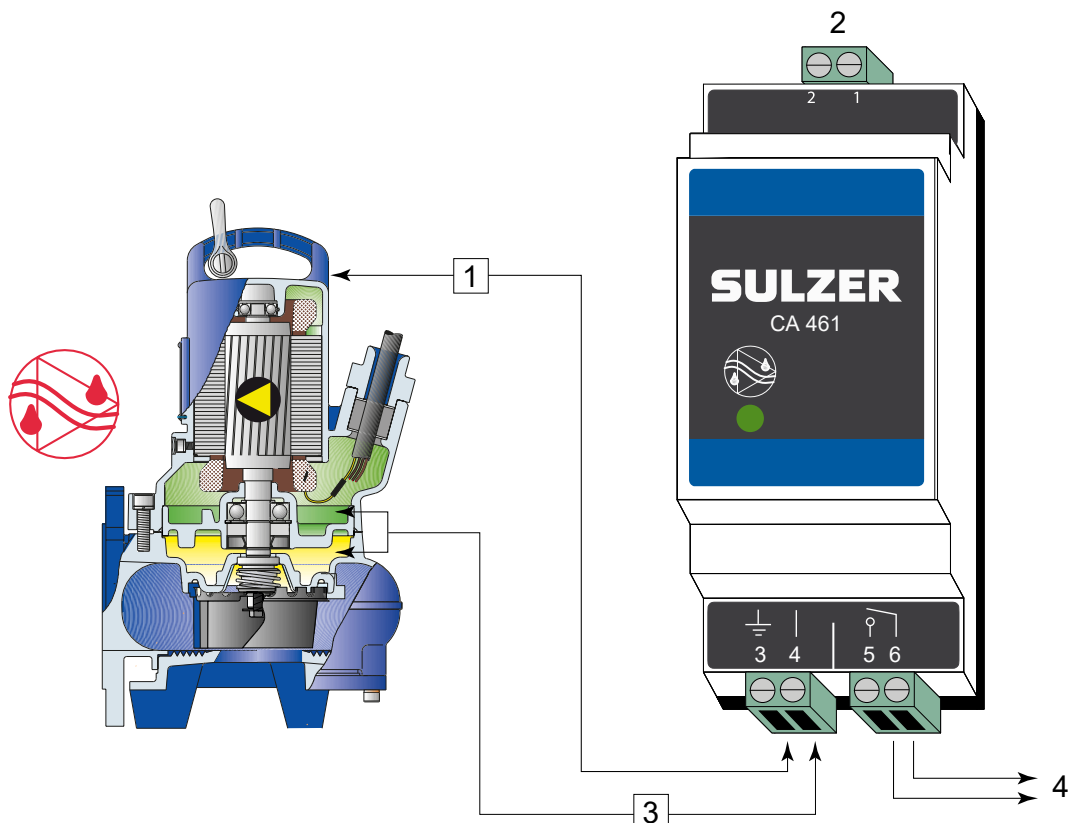
Abbildung 5. Sulzer-Leckageüberwachung Typ CA 461
