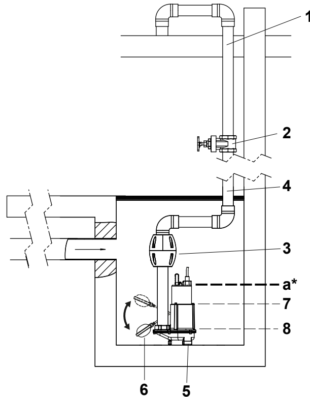
Figur 2: Installeringsseksempel, pumpekum i betong
